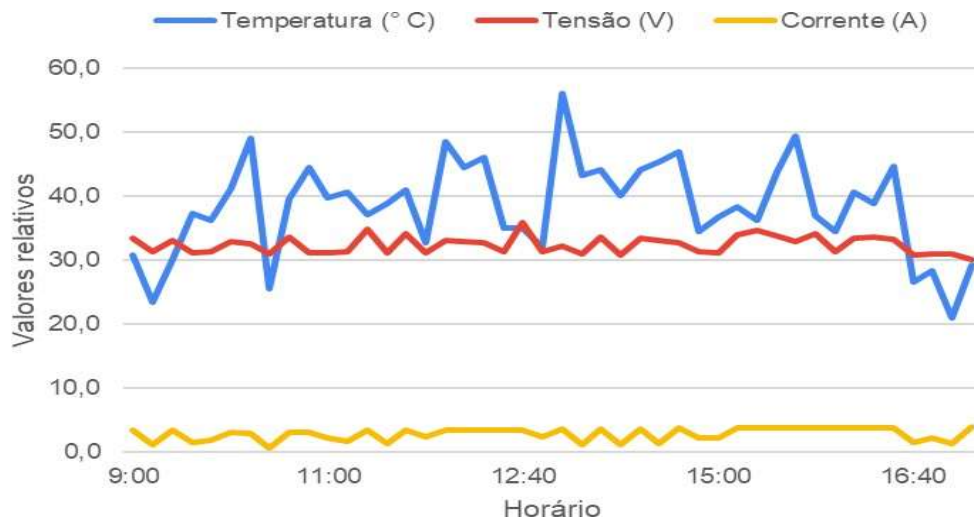
FIGURA 1 . Valores médios observados ao longo dos dias, de Temperatura ( ° Celsius - C), tensão elétrica ( volts -V), corrente elétrica (Amperes – A), em função do horário de coleta.
