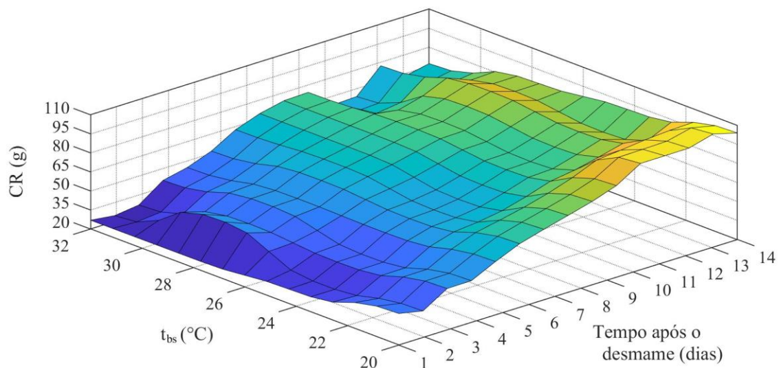
FIGURA 2 - Superfície de resposta do consumo de ração (CR, g) em função da temperatura de bulbo seco do ar ( t_{bs} , °C) e do tempo após o desmame (dias) de coelhos Nova Zelândia Branco.
