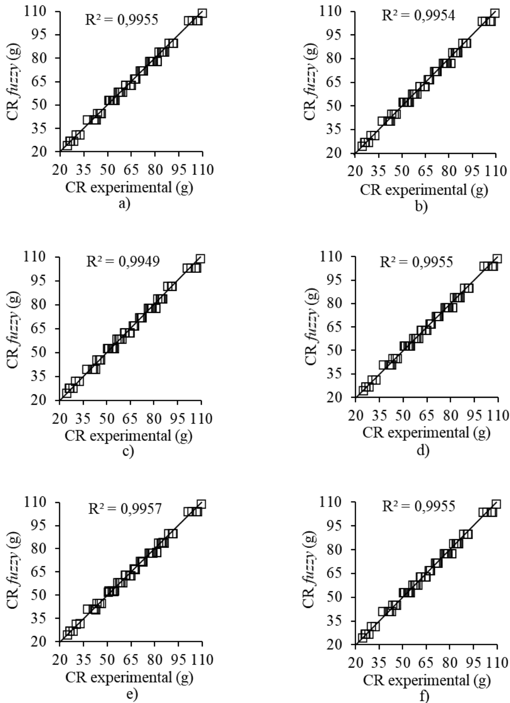
FIGURA 1. Relação funcional entre os valores de consumo de ração obtidos experimentalmente (CR experimental) e preditos pelos sistemas fuzzy (CR fuzzy ), para funções (a) triangulares para defuzzificação mom , (b) gaussianas e defuzzificação lom , (c) trapezoidais e defuzzificação bissetor, (d) triangulares para defuzzificação wsum , e) gaussianas para defuzzificação wtauer , f) trapezoidais e defuzzificação wsum .
