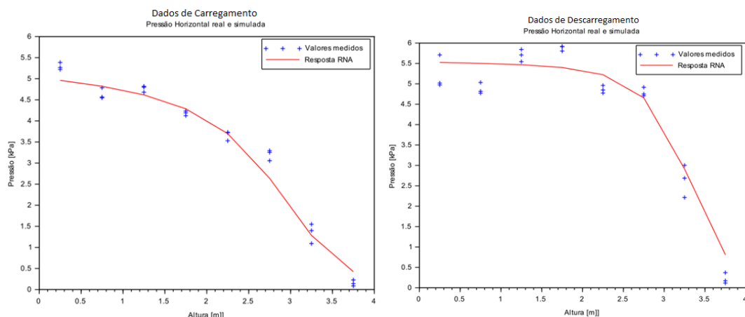
Figura 4. Variação das pressões normais de carregamento e descarregamento
