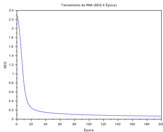
Figura 3. Variação do erro em relação ao número de épocas
