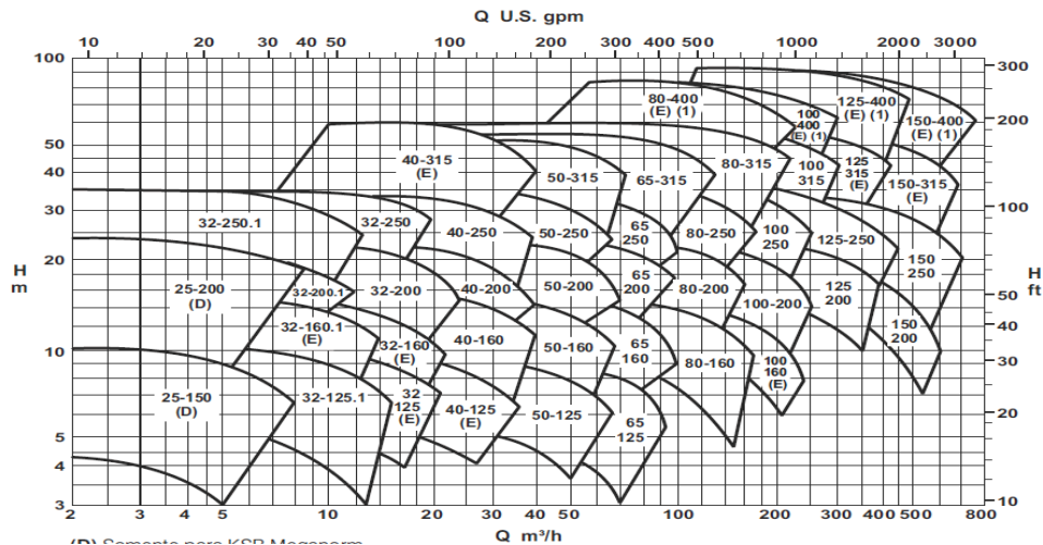
FIGURA 3. Gráfico da curva das bombas KSB MegaNorm 1750rpm (KSB, 2013).
