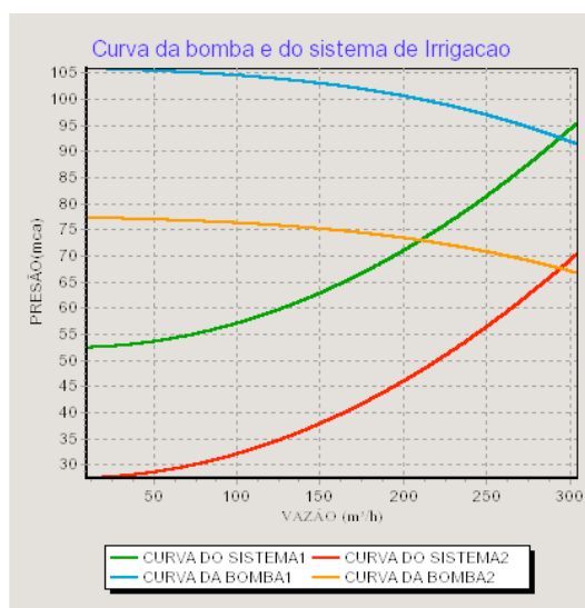
FIGURA 5. Gráfico da curva da bomba e do sistema de irrigação com e sem controle.
