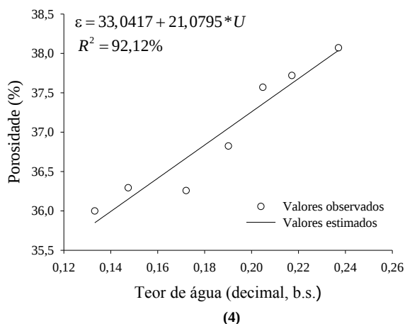
Figura 4. Valores observados e estimados de porosidade intergranular em função do teor de água.
