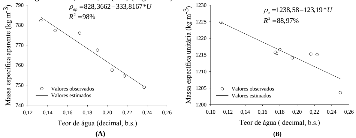
Figura 3. Valores observados e estimados da massa específica aparente (A) e da massa específica unitária (B) dos grãos de feijão caupi em função do teor de água (decimal, b.s.).
