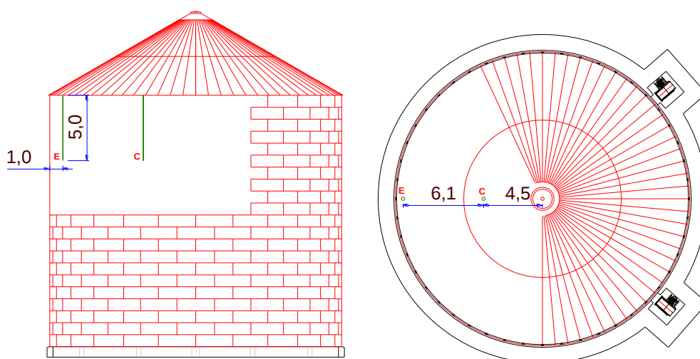
FIGURA 1. Corte e vista superior de um silo, demonstrando as posições de coleta das amostras (medidas em metros).
