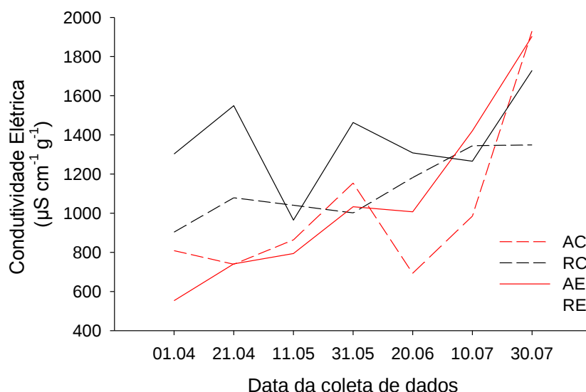
FIGURA 5. Valores observados de condutividade elétrica da solução de exsudatos dos grãos de soja obtidos do centro (C) e extremidade (E) dos silos com aeração com ar natural (A) e sob refrigeração (R) durante o armazenamento. Sinop – MT, 2015.
