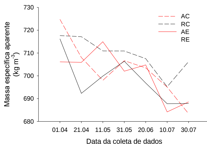
FIGURA 4. Valores observados de massa específica aparente de grãos de soja obtidos do centro (C) e extremidade (E) dos silos com aeração com ar natural (A) e sob refrigeração (R) durante o armazenamento. Sinop – MT, 2015.
