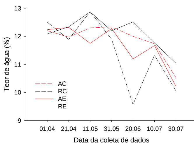
FIGURA 3. Valores observados do teor de água de grãos de soja obtidos do centro (C) e extremidade (E) dos silos com aeração com ar natural (A) e sob refrigeração (R) durante o armazenamento. Sinop – MT, 2015.
