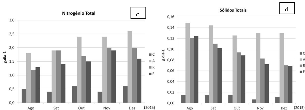
FIGURA 2: Carga (g.dia -1 ) de DQO (a), COT (b), NT (c) e ST (d) de agosto a dezembro de 2015 nos pontos C, A, R e F.
