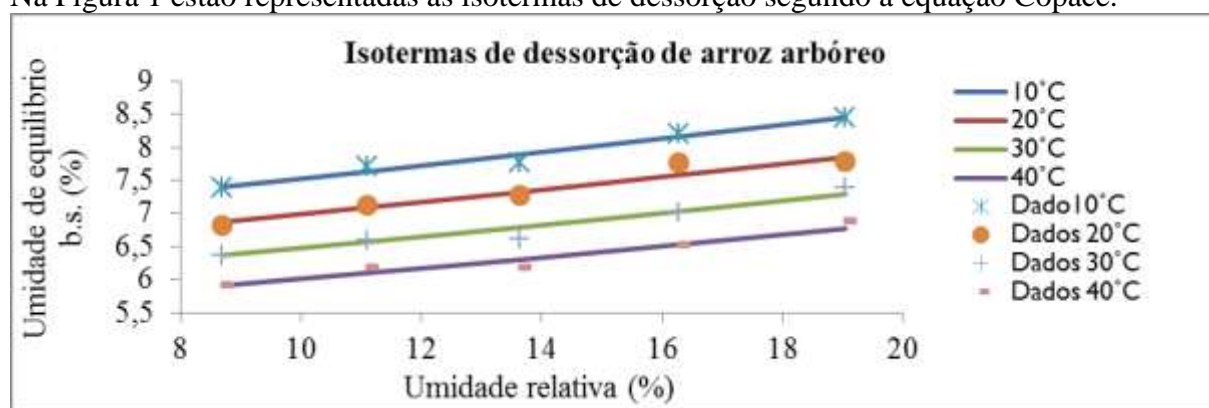
Figura 1. Isotermas de dessecção de arroz arbóreo segundo o modelo matemático Copace e dados experimentais
