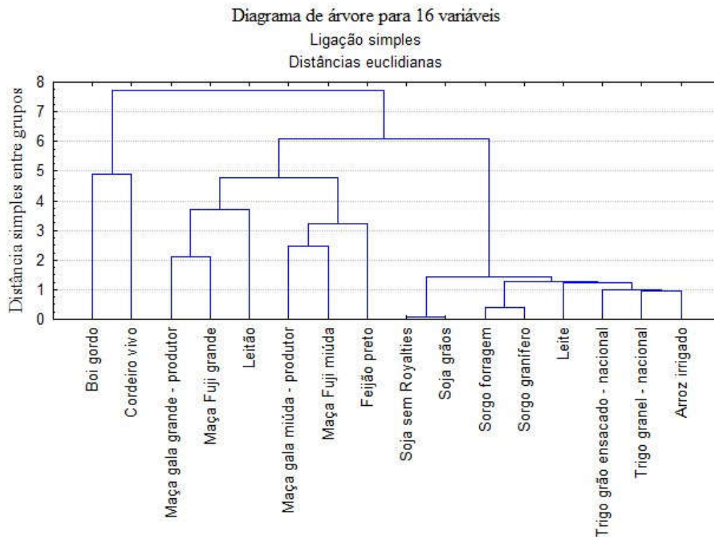
Figura 1 – Dendrograma das 16 variáveis feito por ligação simples e distancias euclidianas.
