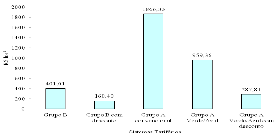
Figura 2. Estimativa do custo do consumo de energia elétrica (CCEE), para os sistemas tarifários estudados.
