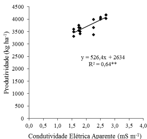
FIGURA 2. Regressão entre a produtividade da soja e a condutividade elétrica aparente do solo. Regression for soybean yield and soil electrical conductivity.
