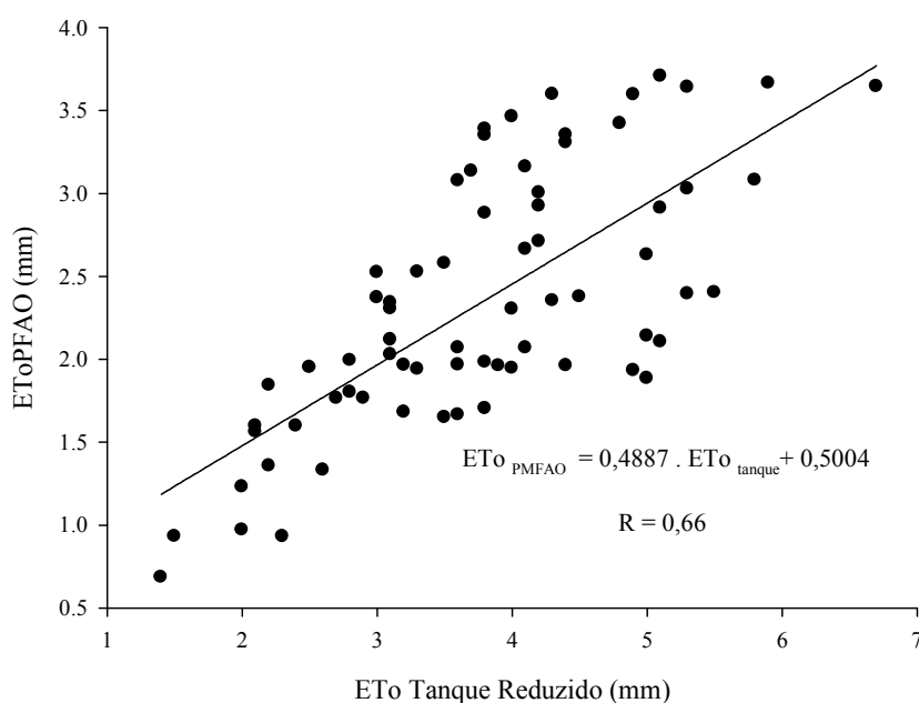
FIGURA 2. Gráfico das ET 0 Tanque reduzido pela ET 0 Penman-Monteith
